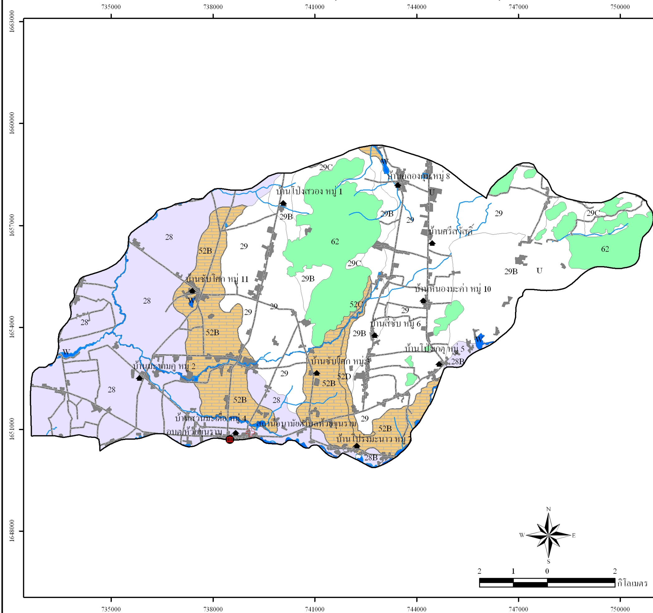
รูปที่ 3-1 แผนที่ทรัพยากรดิน ตำบลห้วยขุนราม อำเภอพัฒนานิคม จังหวัดลพบุรี
